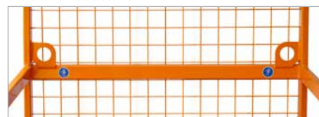
Anschlagpunkte für PSA (Persönliche Schutzausrüstung)
