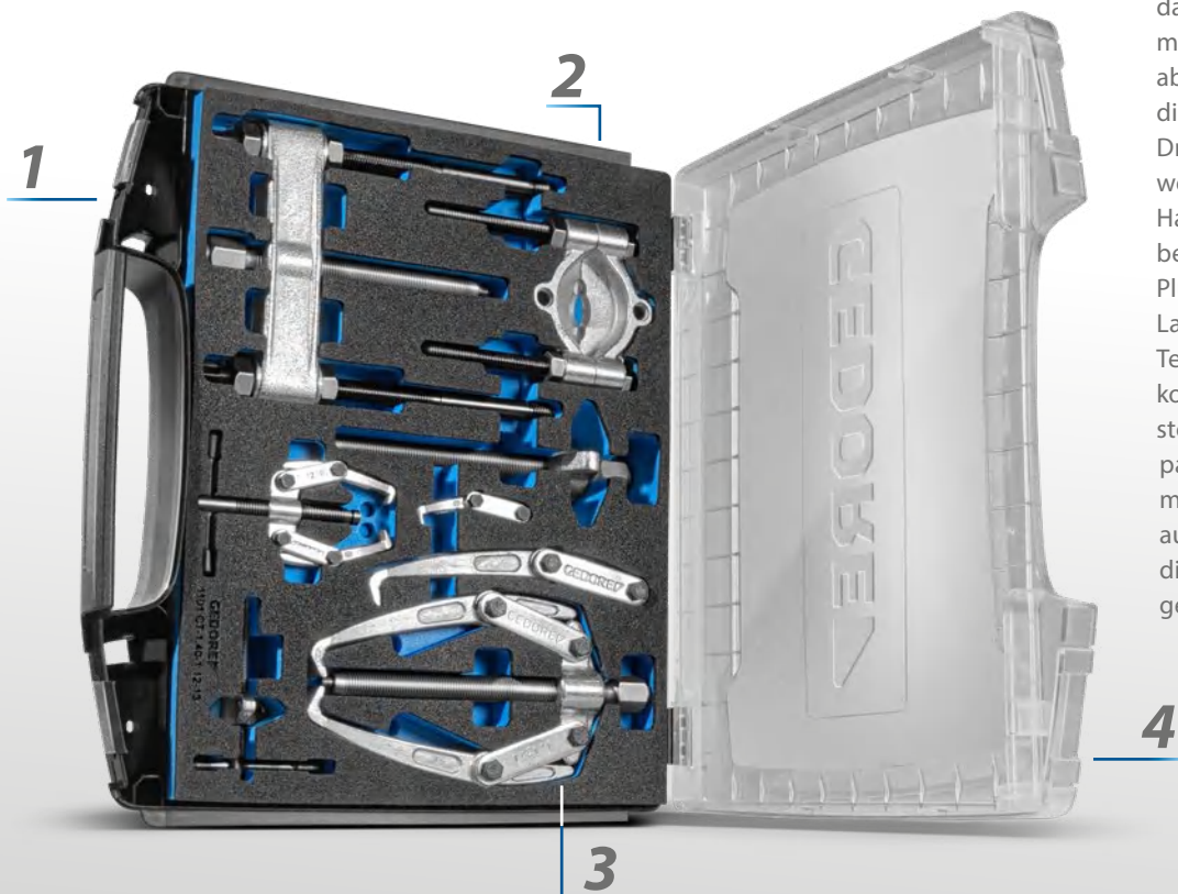
Trenn- und Abzieher-Set zwei- und drei-armig 1101-1.40-1.12-13
